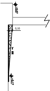
Corte A - B Escala: 1:25
