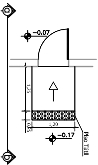
Planta Baixa Escala: 1:50
