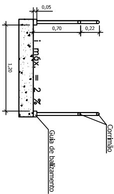
Detalhe transversal da rampa Escala: 1:25
